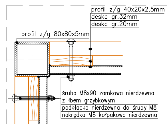
DETAL 2: PANEL DREWNIANY – ŁĄCZENIE 1:5
