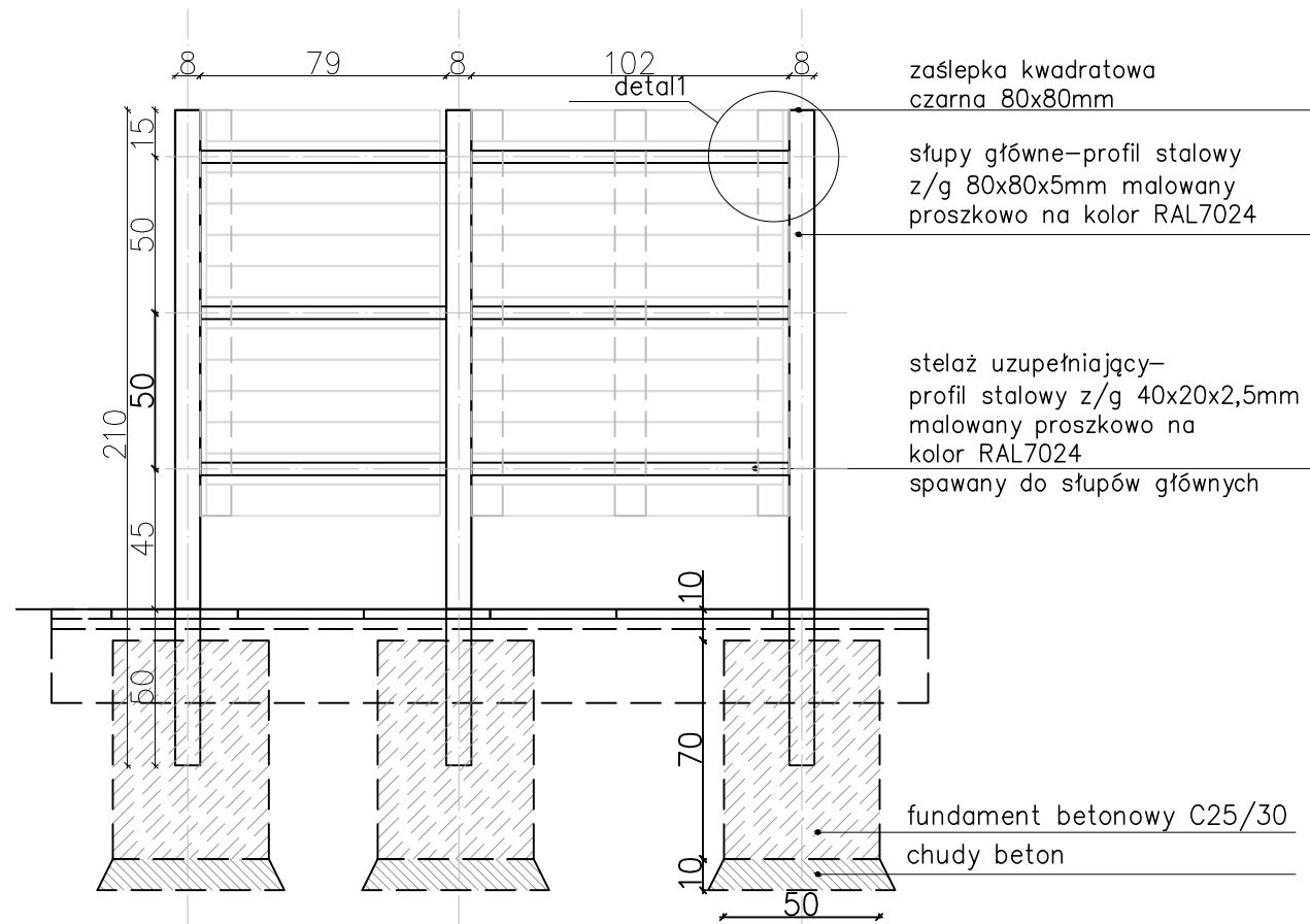
PRZEBIERALNIA (OZN.6) WIDOK – KONSTRUKCJA 1:25
