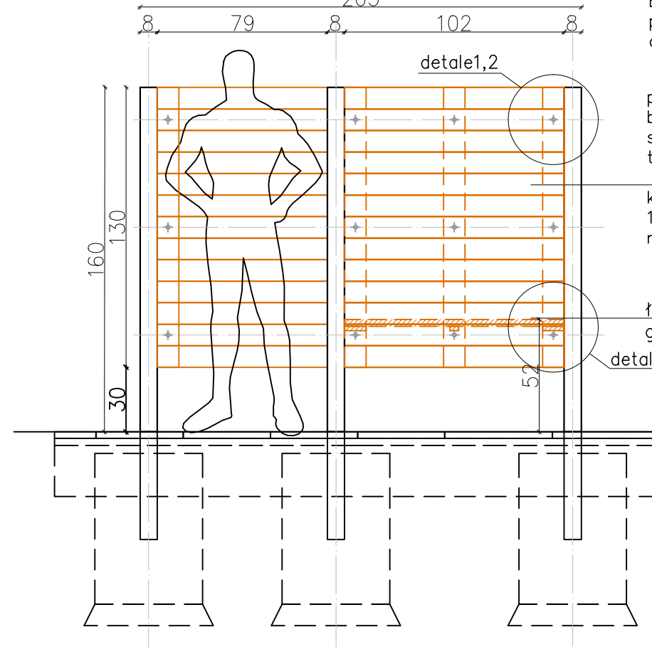
PRZEBIERALNIA (OZN.6) WIDOK – DESKOWANIE 1:25
