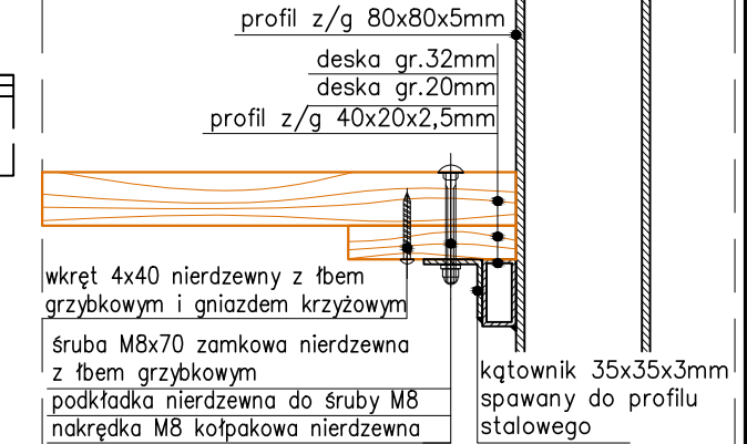
DETAL 3: MONTAŻ ŁAWKI/PÓŁKI 1:5
