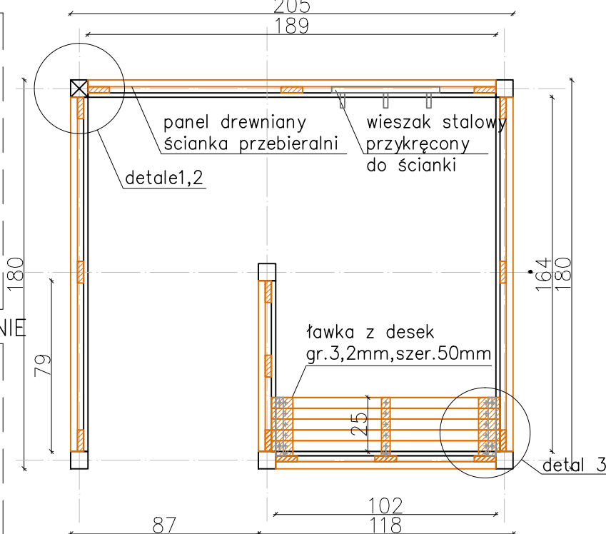
PRZEBIERALNIA (OZN.6) DESKOWANIE – RZUT 1:25
