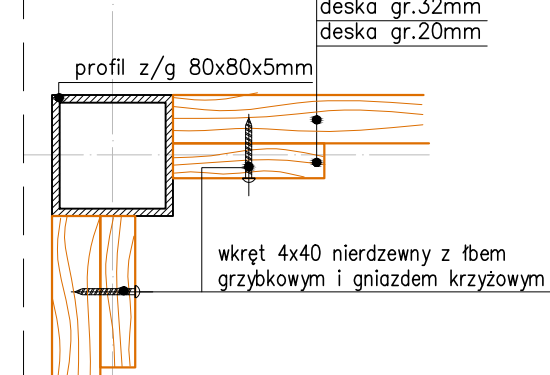
DETAL 2: PANEL DREWNIANY – ŁĄCZENIE 1:5
