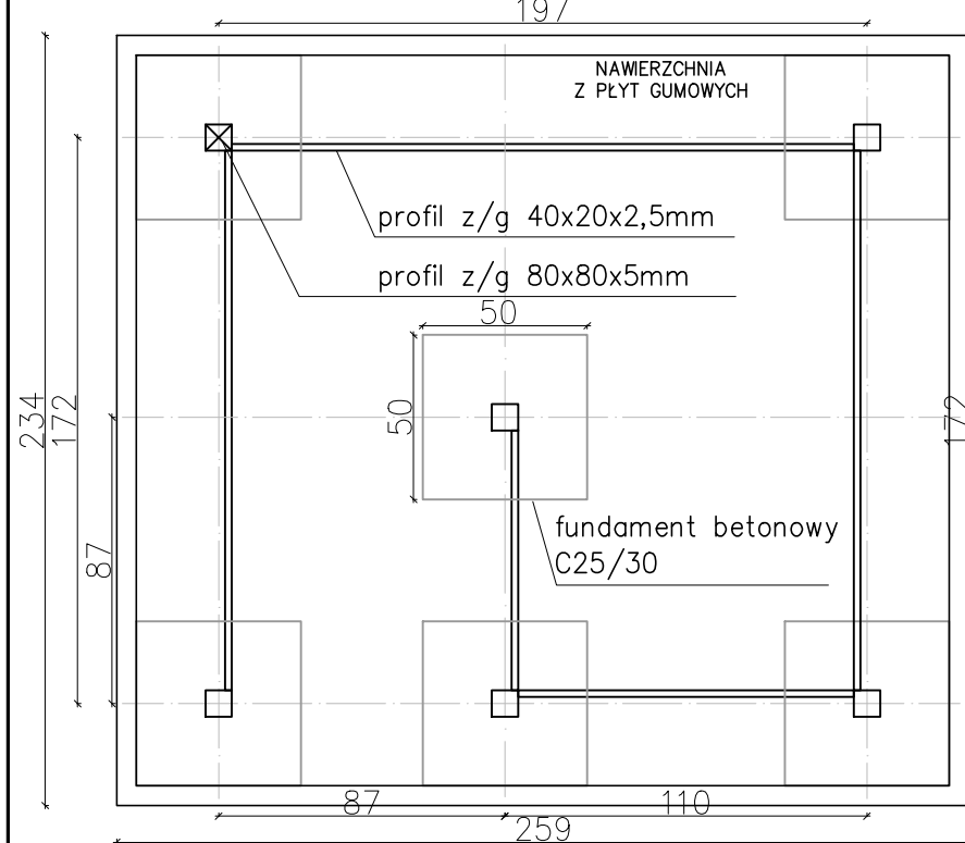
PRZEBIERALNIA (OZN.6) GEOMETRIA – RZUT 1:25
